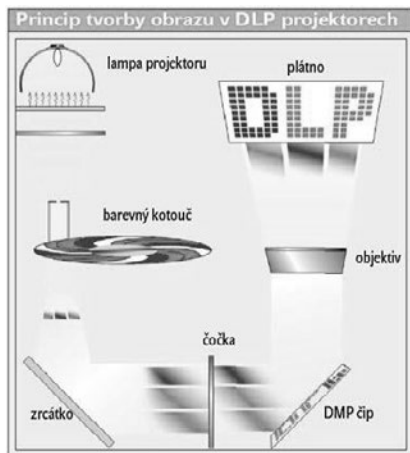
Obrázek 1.7: Schéma DLP projektoru
